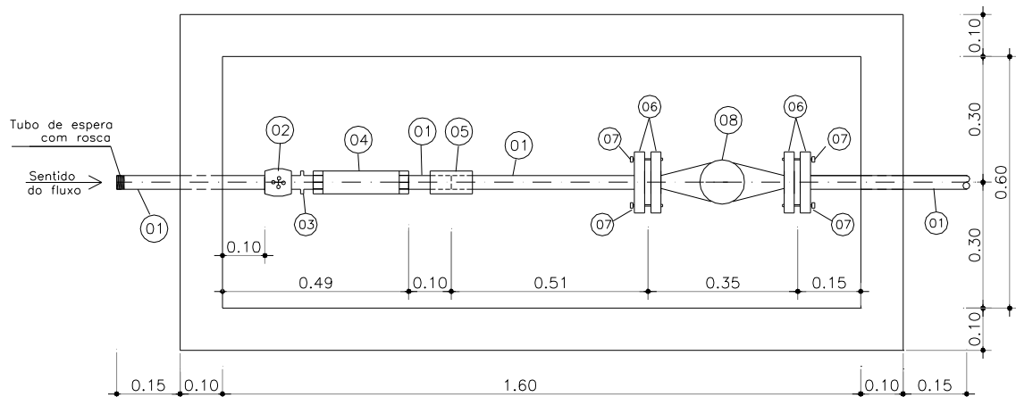
VISTA SUPERIOR
