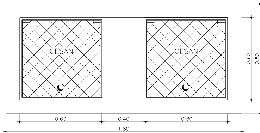
VISTA SUPERIOR
