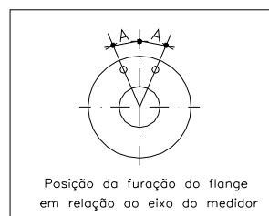
DETALHE DO FLANGE
