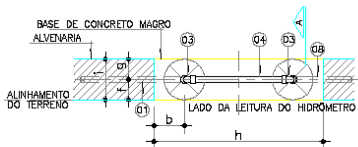
PLANTA BAIXA
