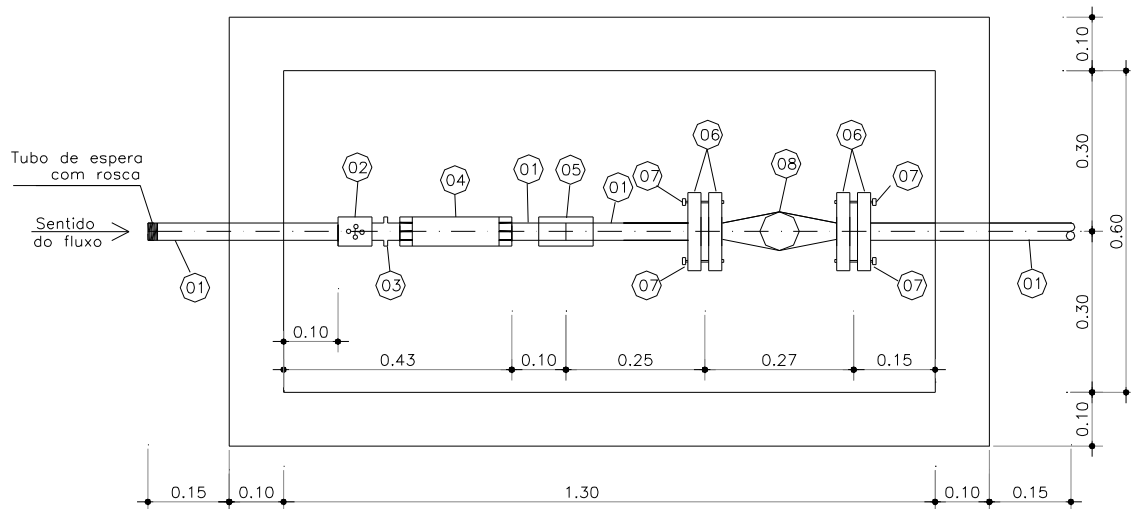
VISTA SUPERIOR COM HIDRÔMETRO
