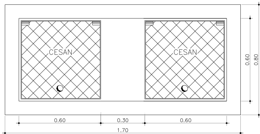
TAMPA TIPO 3
