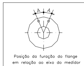
DETALHE DO FLANGE
