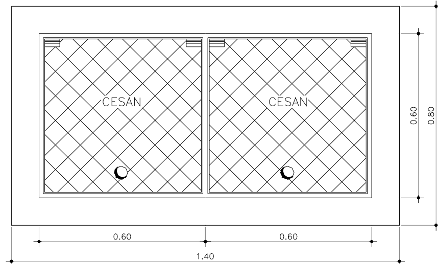
VISTA SUPERIOR COM HIDRÔMETRO
