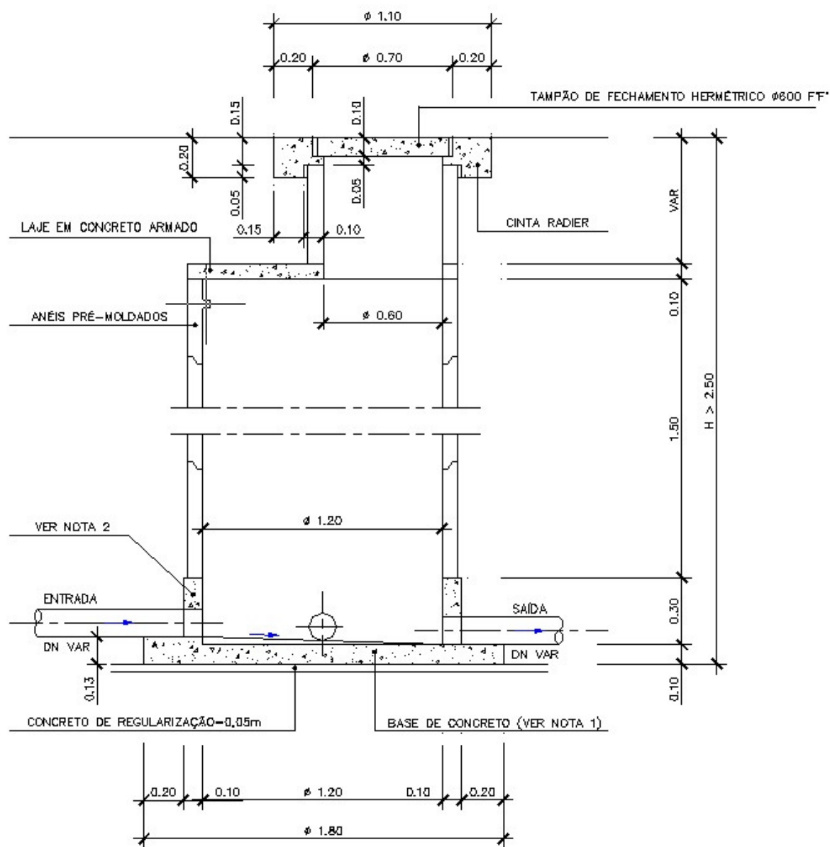
CORTE-AA'
