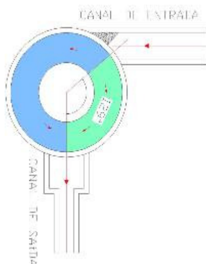
FIGURA 2. MECANISMO DE SEDIMENTAÇÃO HORIZONTAL NO DESARENADOR DO TIPO VÓRTEX.
