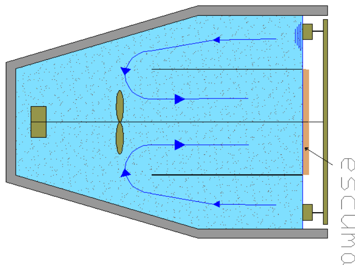
FIGURA 6. SITUAÇÃO ATUAL DO DESARENADOR EXISTENTE.
