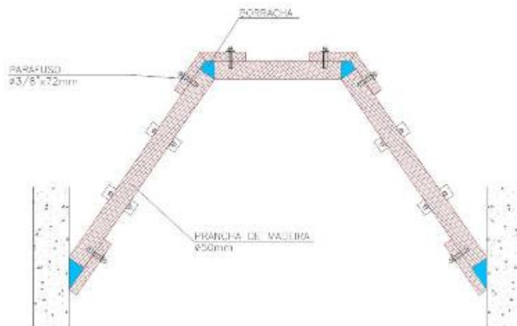
FIGURA 10. DETALHE 1 - VISTA SUPERIOR DO ESQUEMA DE INSTALAÇÃO DAS PRANCHAS DE MADEIRA.
