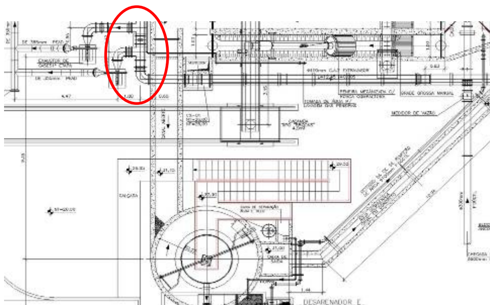
FIGURA 7. FECHAMENTO DA COMPORTA DO CANAL DE ENTRADA DO DESARENADOR.
