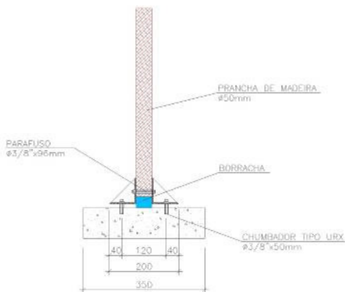
FIGURA 11. DETALHE 2 - FIXAÇÃO DAS PRANCHAS NO FUNDO DO CANAL.
