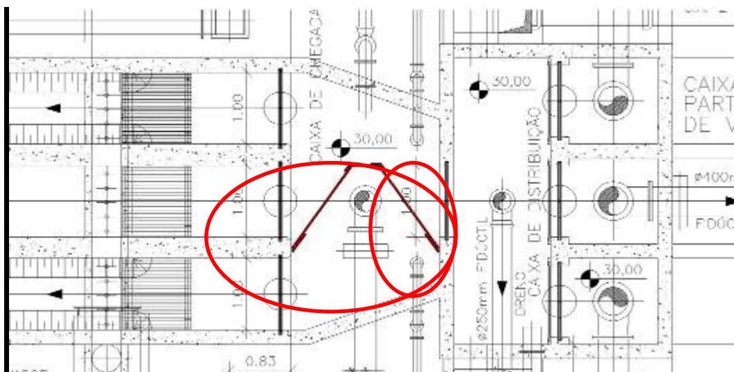
FIGURA 9. INSTALAÇÃO DE PRANCHAS DE MADEIRA COM VEDAÇÃO E ABERTURA DA COMPORTA ENTRE A CAIXA DE CHEGADA E A CAIXA DE DISTRIBUIÇÃO.
