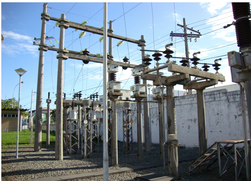
Fotos 1 e 2 – Vista Geral da Subestação
