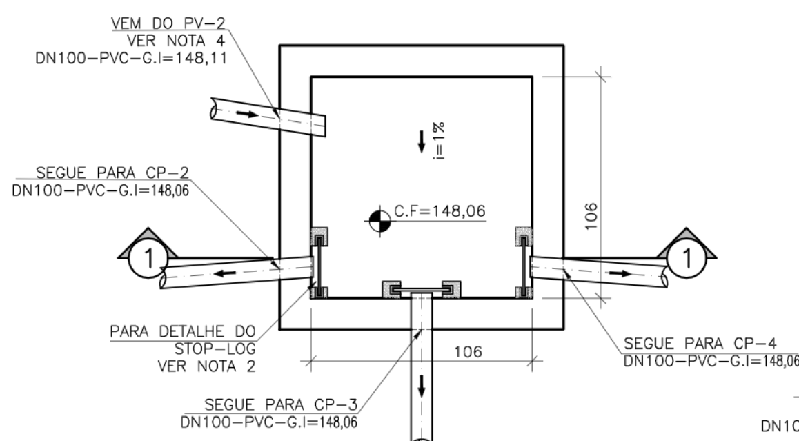
PLANTA CP1 ESCALA: 1/25
