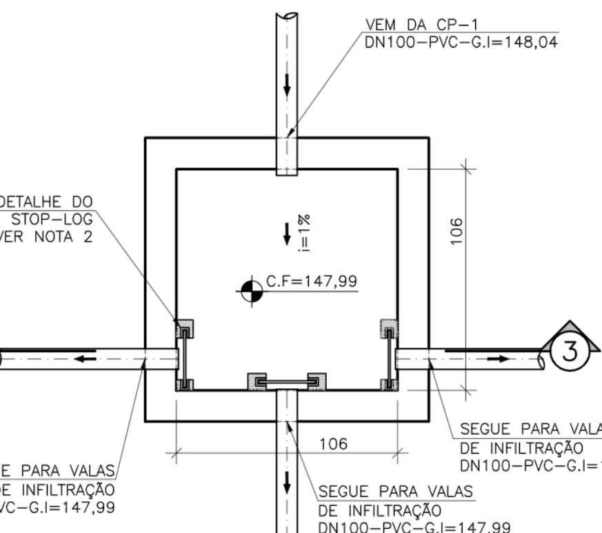
PLANTA CP3 ESCALA: 1/25
