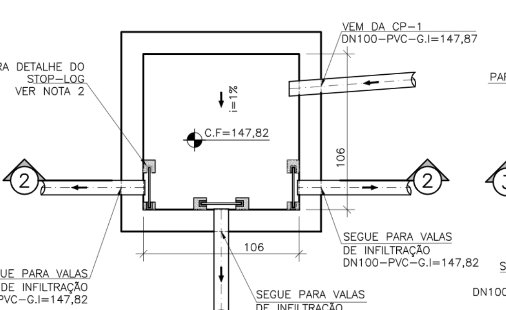
PLANTA CP2 ESCALA: 1/25
