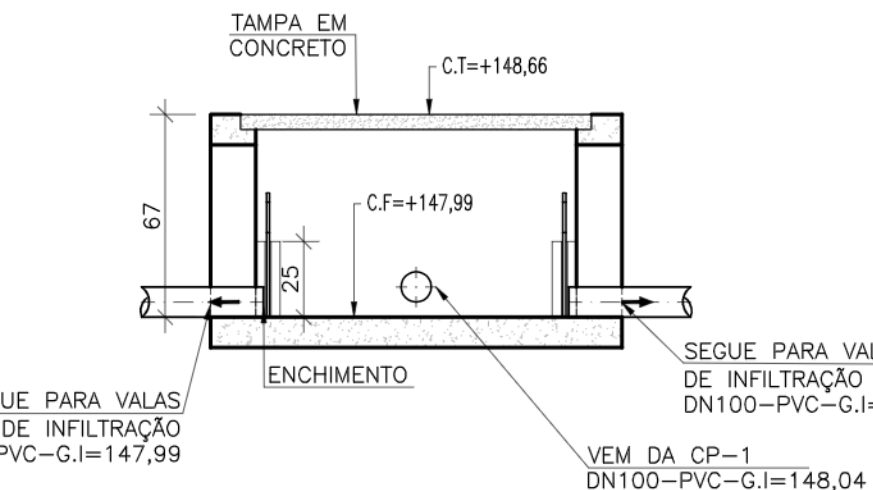
CORTE 3-3 CP3 ESCALA: 1/25
