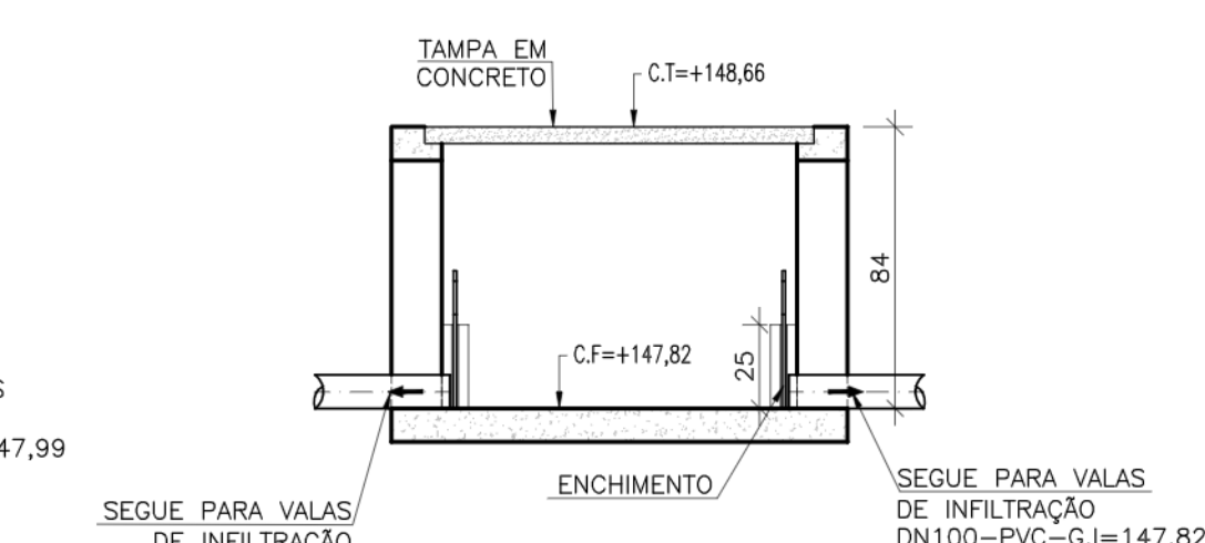
CORTE 4-4 CP4 ESCALA: 1/25
