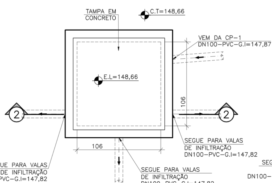
VISTA SUPERIOR CP2 ESCALA: 1/25
