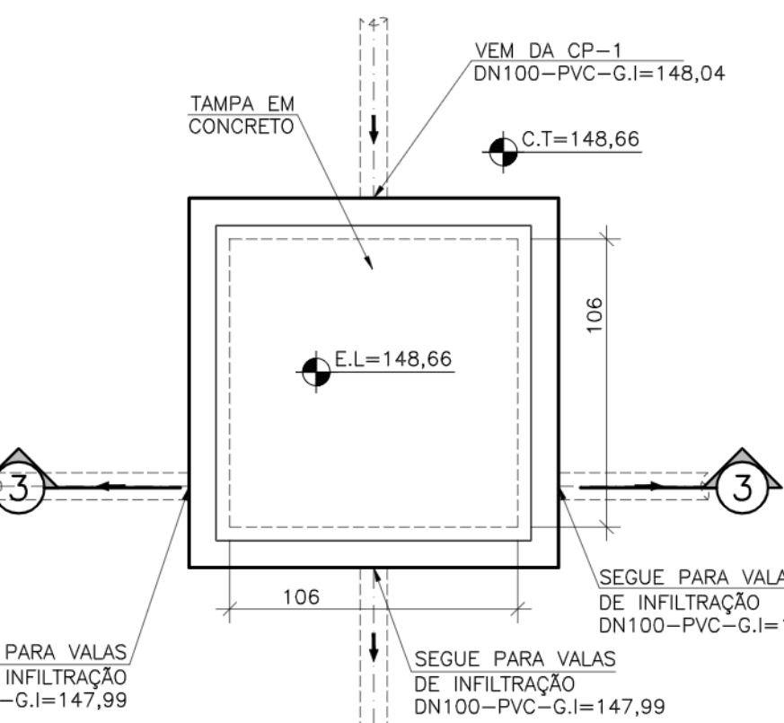
VISTA SUPERIOR CP3 ESCALA: 1/25
