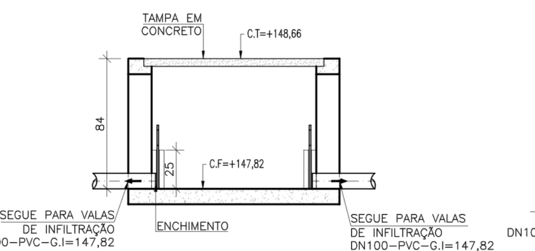
CORTE 2-2 CP2 ESCALA: 1/25
