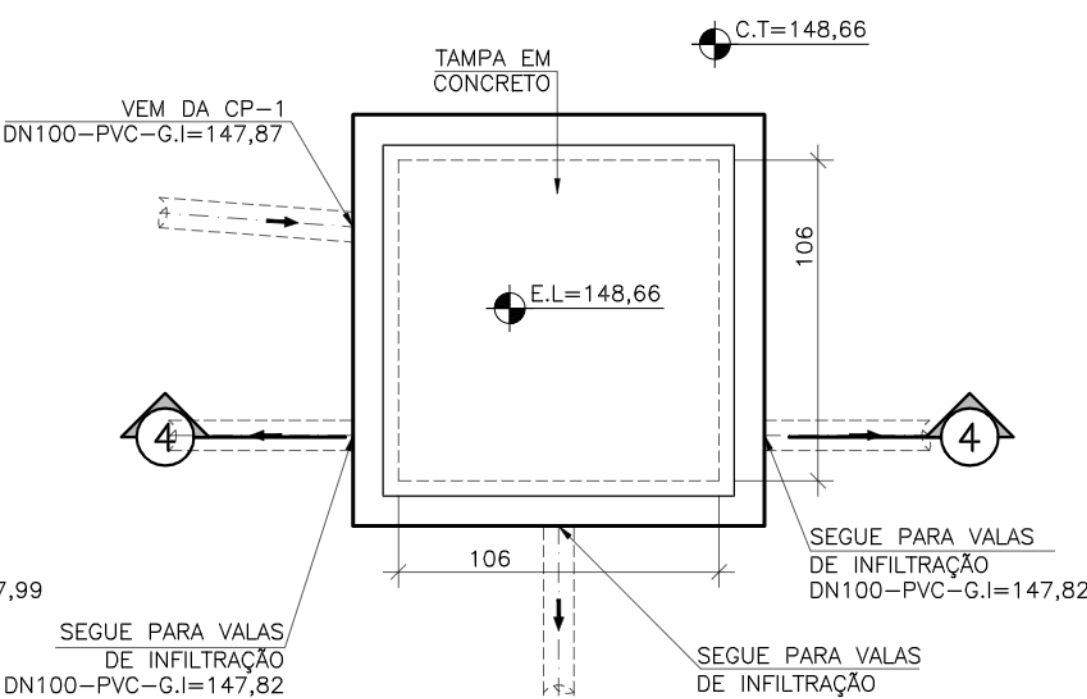
VISTA SUPERIOR CP4 ESCALA: 1/25
