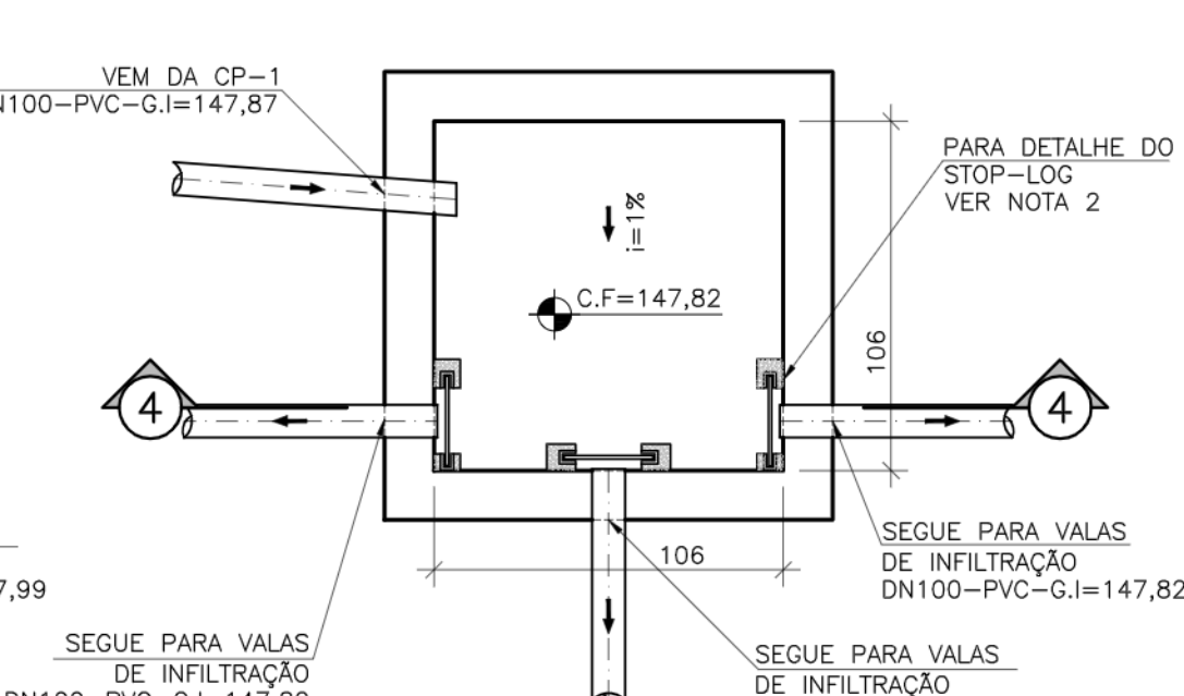
PLANTA CP4 ESCALA: 1/25
