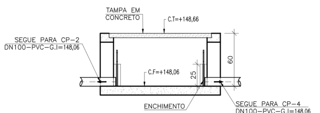
CORTE 1-1 CP1 ESCALA: 1/25
