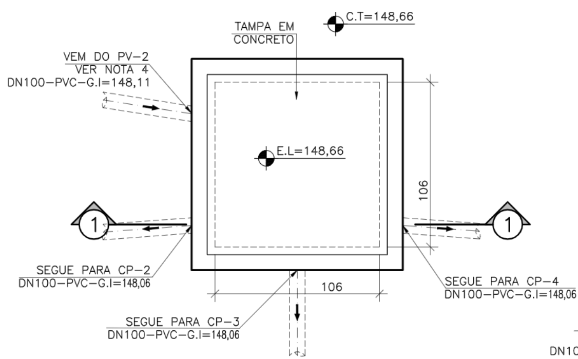
VISTA SUPERIOR CP1 ESCALA: 1/25
